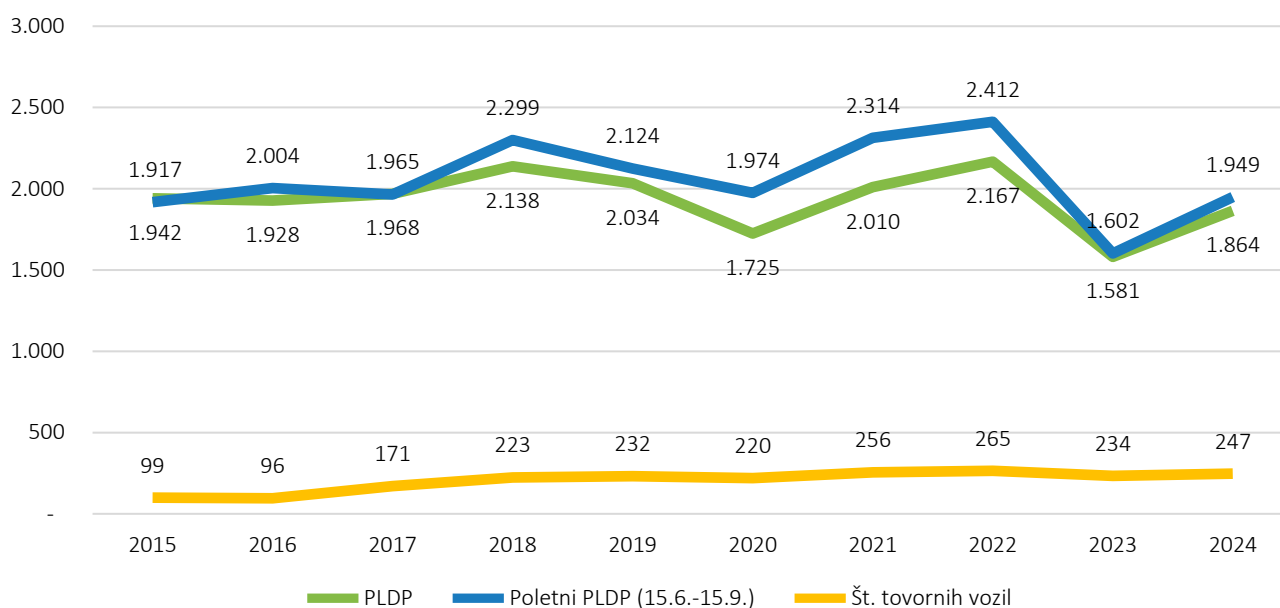
Gibanje količine prometa na avtomatskem števnem mestu 264 Horjul v obdobju 2016–2024.
